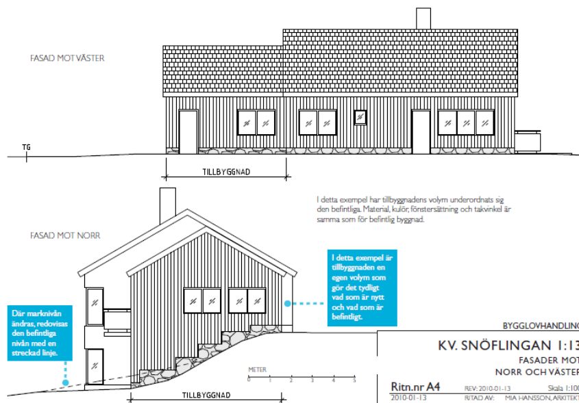
Figur 1 Exempel på hur en fasadritning ser ut
