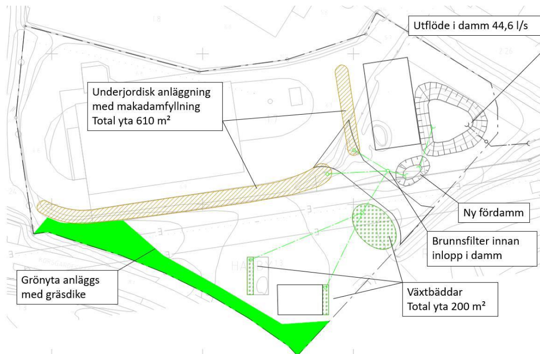
Figur 23. Föreslagen dagvattenhantering inom planområdet. (Dagvattenutredningen)
