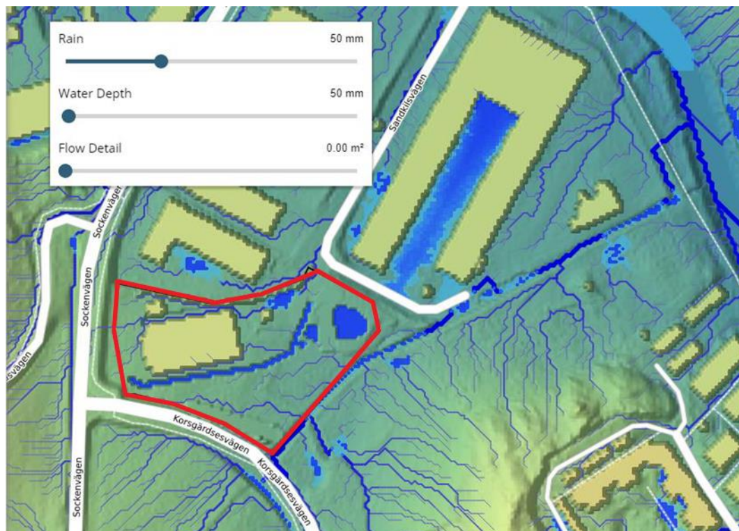
Figur 19. Översvämmade områden med vattendjup mer än 50 mm i befintlig situation är markerade med blått. Plangränsen är markerad med röd linje. (Dagvattenutredningen)
