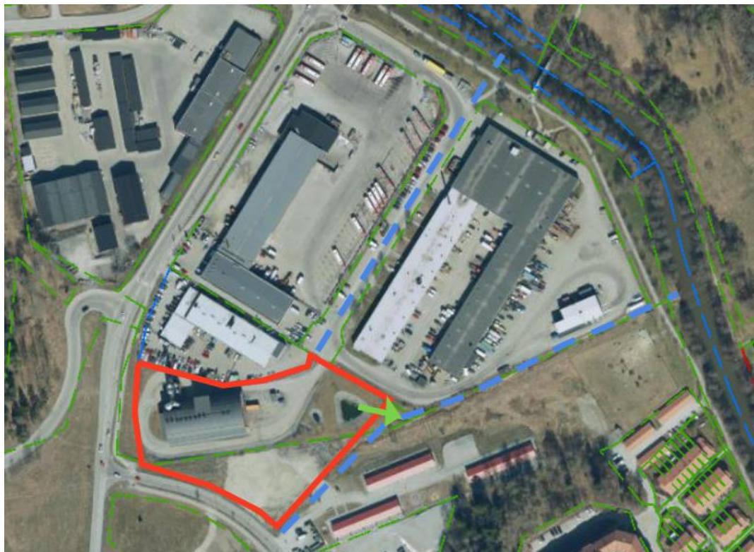
Figur 22. Befintliga avrinningsvägar för skyfall från planområdet markerat med blå streckad linje. (Dagvattenutredningen)
