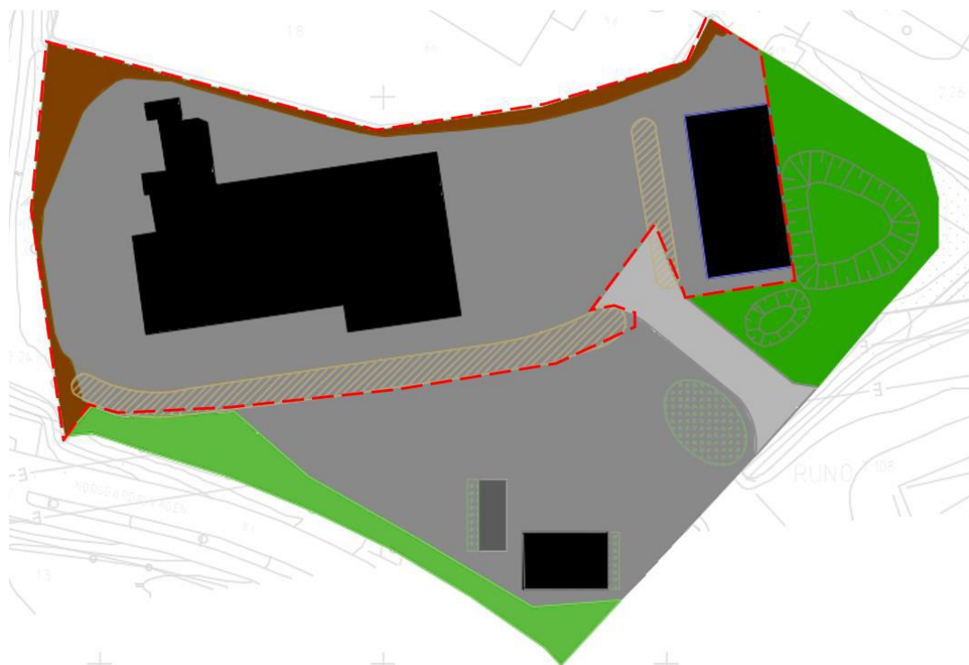
Figur 25. Ytor som avleds till makadammagasin är inringade med röd streckad linje. (Dagvattenutredningen)
