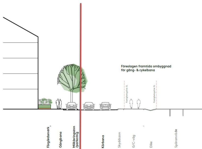
Figur 18. Föreslagna ny gatusektion för Västra Banvägen vid aktuell fastighet som tagits fram i samband med arbetet för denna detaljplan. Plangränsen till aktuell detaljplan illustreras med en röd
