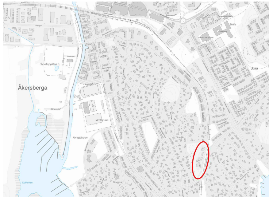
Översiktskarta
