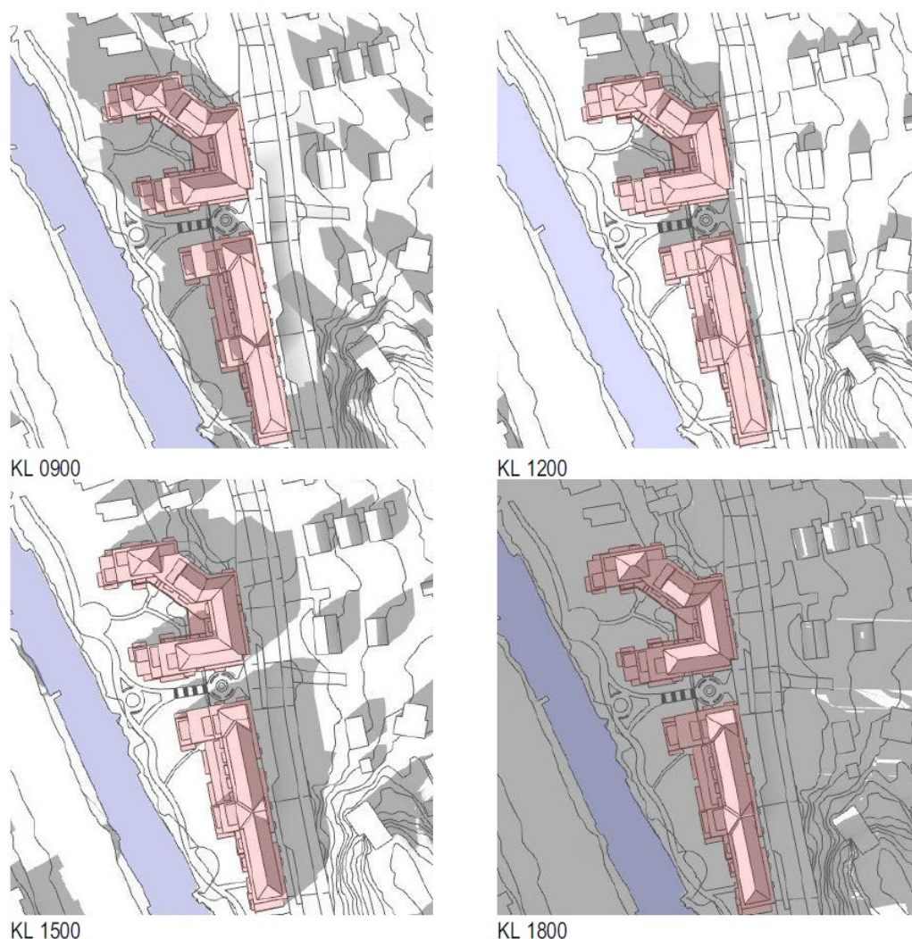
Figur 20. Solstudie höst- och vårdagjämning för bebyggelsen i norra delen av Kanalterrassen.
