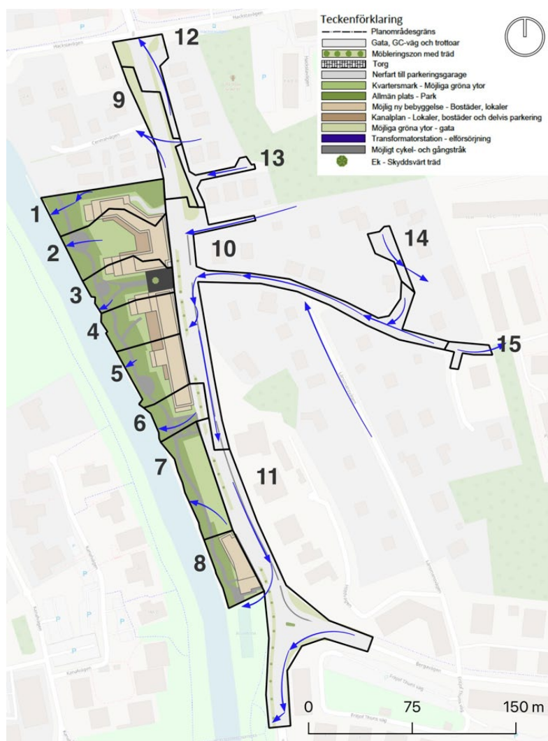
Figur 24. Planområdet indelat i avrinningsområden för framtida markanvändning. Blå pilar anger huvudsakliga flödesvägar för ytvatten (Dagvattenutredning för Kanalterrassen, 2023). Flödesvägar är reviderade efter uppdaterad höjdsättning av gata enligt redovisad bild.
