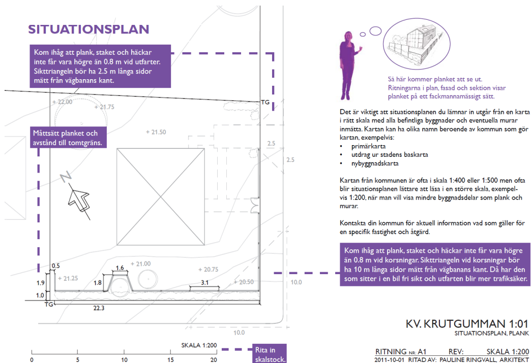
Figur 1 Exempel på en situationsplan
