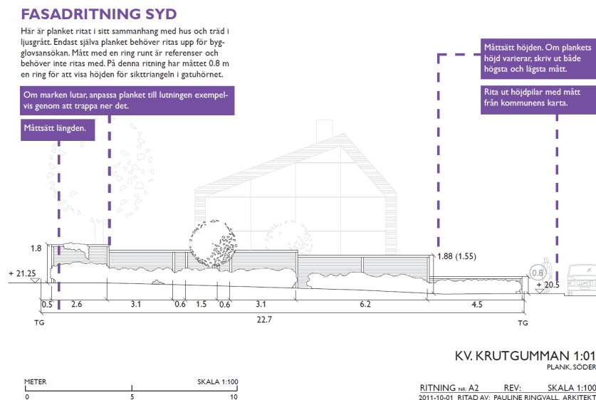
Figur 2 Exempel på fasadritning
