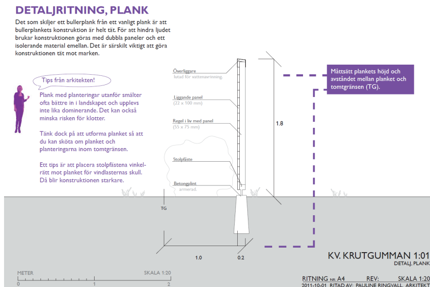
Figur 3 Exempel på detaljrättning
