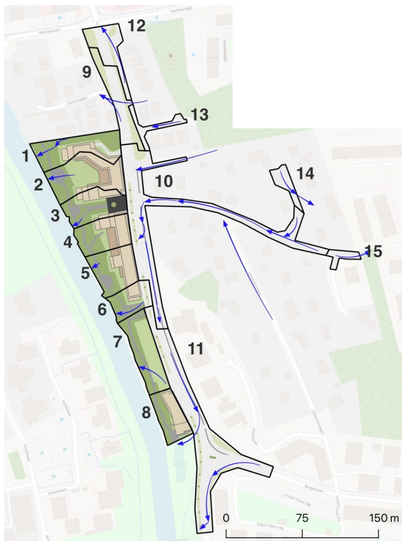
Figur 23. Planområdet indelat i avrinningsområden för framtida markanvändning. Blå pilar anger huvudsakliga flödesvägar för ytaavrinning (Dagvattenutredning för Kanalterrassen, 2023). Flödesvägar är reviderade efter uppdaterad höjdsättning av gata enligt redovisad bild.
