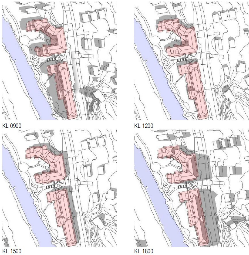
Figur 18. Solstudie sommarsolstånd för bebyggelsen i norra delen av Kanalterrassen.
