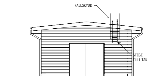
FASAD MOT SYDVÄST_FRD 1 : 100
