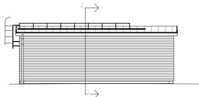
FASAD MOT SYDÖST_FRD 1 : 100
