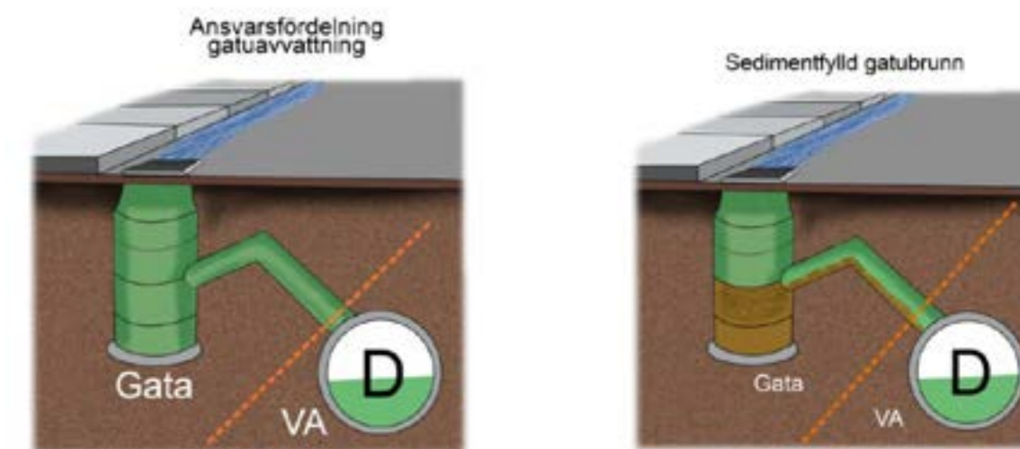
Figur 3. Schematisk bild över ansvarsfördelning av dagvatten, mellan gata (vaghållare, ex. vägförening eller kommun) och VA-huvudman avseende gatans avvattning (ur VAV P110 Svenskt Vatten).
