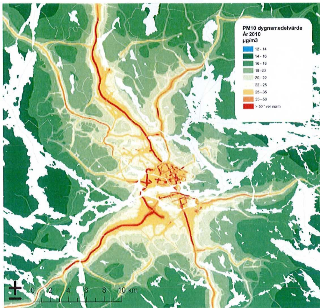
Figur 2.9. PM 10 2010, dygnsmedelvärde mikrogram/m 3 . Rött illustrerar överskridande av miljö kvalitetsnorm (MKN) över 50 mikrogram/m 3 . Gult indikerar att MKN kan överskridas. Måttet ur hälsosynpunkt är 30 mikrogram/m 3 .
