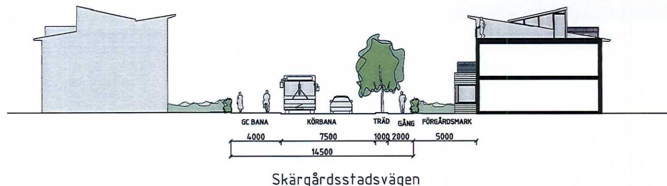
Sektion av bebyggelse tvärs Skärgårdsstadsvägen med det gaturum förslaget framhäver där Skärgårdsstadsvägen ska uppfattas mer som en lokalgatan än.
