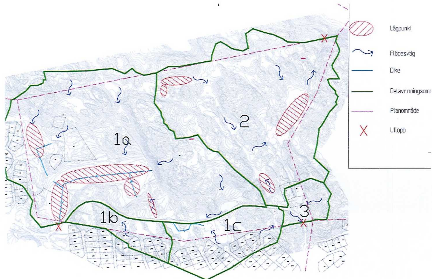
Programområdets avrinningsområde indelat i delområden. Lågpunkter, rinnvägar, diken samt utlopp från delområde visas i illustrationen.
